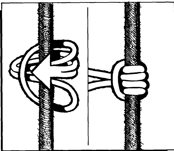
Figure 22-9. Prusik Knot.
