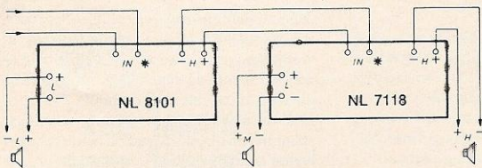
Aansluitschema van de twee scheidsfilters voor driefwagsystemen met een hoge belastbaarheid.
