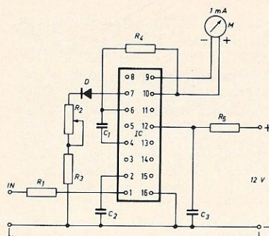
Schema van de nieuwe tachometer NL 1822 met geïntegreerde schakeling.
