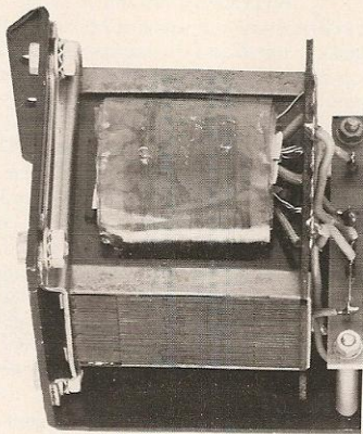
Een voedingstransformator waarbij alle spoelen om het „middenbeen” van de ijzern kern zijn gewikkeld.
