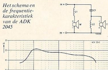
Het schema en de frequentie-karakteristiek van de ADK 2560
