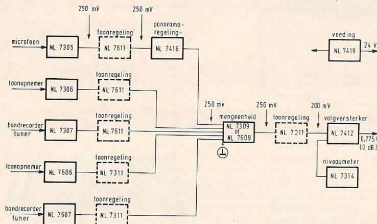
Abbeelding 2. De reeks Philips onderdelenpakketten voor mengversterkers kan op vele manieren worden gecombineerd. De in dit blokschema getekende samenstelling is maar één voorbeeld. In de handleidingen bij de diverse onderdelenpakketten wordt een groter aantal mogelijkheden aangegeven.
