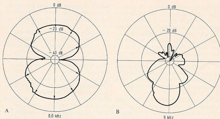
Afb. 6: Stralingsdiagrammen. De lengte van de pijlen is een maat voor de geluidsdruk in die richting.
