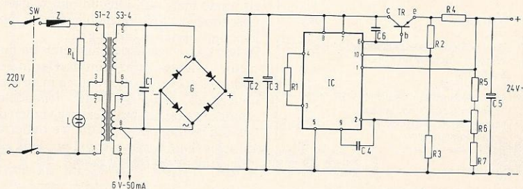
Schema NL 3719
