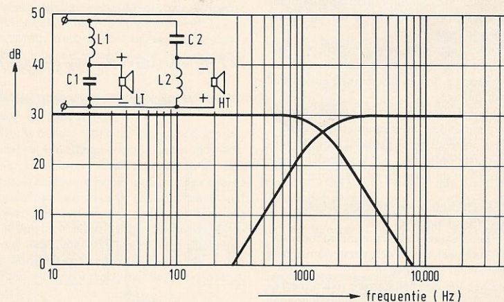
Afb. 5: De scheidingsfrequentie wordt gevormd door het punt waar de frequentiekenarakteristieken van de twee scheidingsfilters elkaar snijden en
