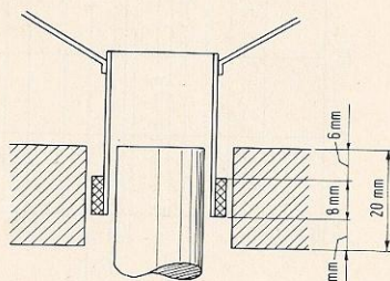
Afb. 2: Een korte spoel in een lange luchtspleet waarborgt een constant magnetisch veld in de spoel.
