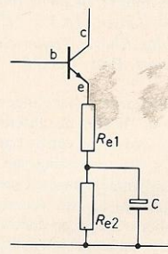
Afb. 10. Tegenkoppeling met „opgedeelde” emitterweerstand.
