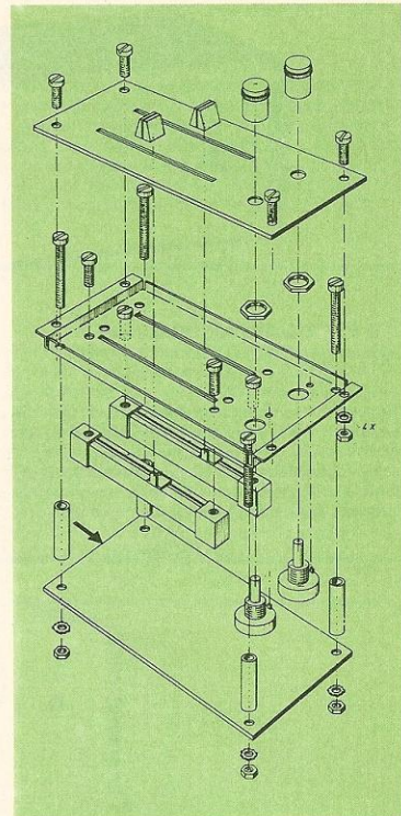
Afbeelding 1. Alle eenheden uit de mengversterkers zijn opgebouwd zoals hier schematisch is weergegeven. De enige uitzondering hierop wordt gevormd door de meng-eenheid NL 7309, die zonder freem en frontplaat wordt geleverd. Van onder naar boven: de printplaat met alle elektronische onderdelen, het freem met schuif- en draaipotentiometers, en de frontplaat met knoppen.
