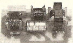
Drieweg luidsprekerscheidingsfilter 500/4000 Hz, 6/6/12 dB NL 4131 (4 Ω), NL 8131 (8 Ω)
