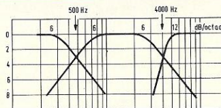
Drieweg luidsprekerscheidingsfilter 500/4000 Hz, 6/6/12 dB NL 4131 (4 Ω), NL 8131 (8 Ω)
